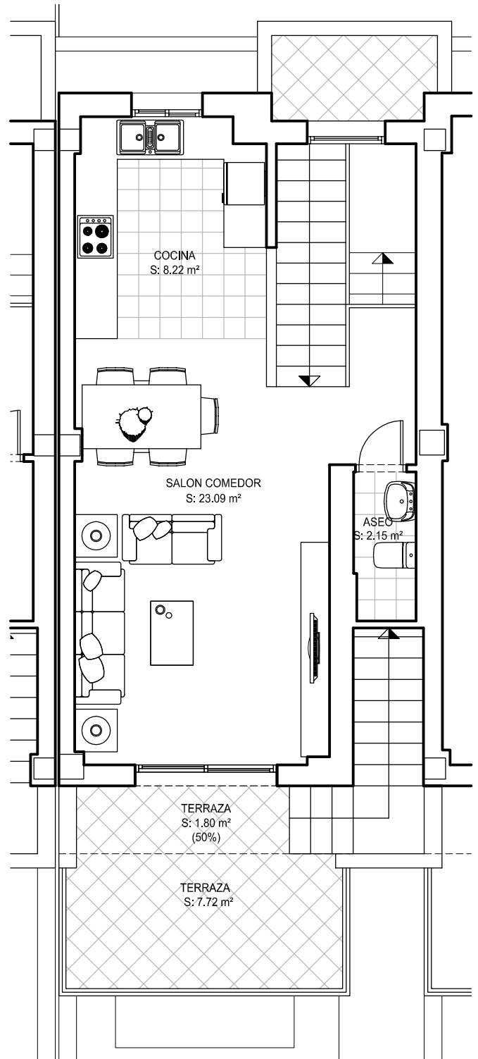
PLANTA ALTA
